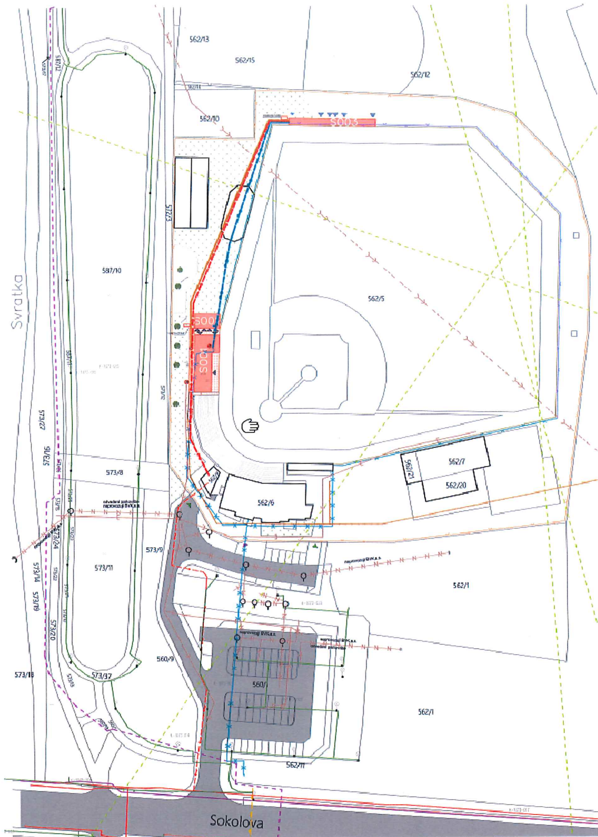
situační výkres
