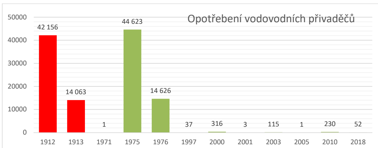
Graf 3: Stav vodovodních přívaděčů v majetku města Brna
