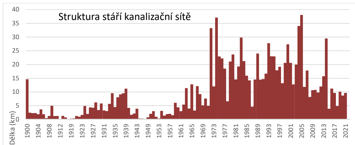
Graf 4: Struktura stáří kanalizační sítě v majetku města Brna
