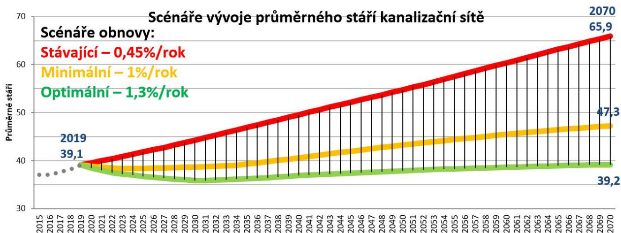
Graf 7: Scénáře vývoje průměrného stáří kanalizační sítě (studie Dlouhodobá strategie obnovy vodovodu a kanalizace , BVK, 2018-2022)
