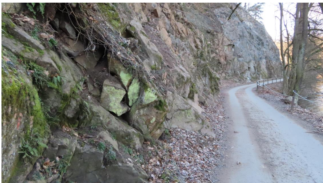
c-V-2 hrozící sesuvy skalních bloků u cyklostezky
