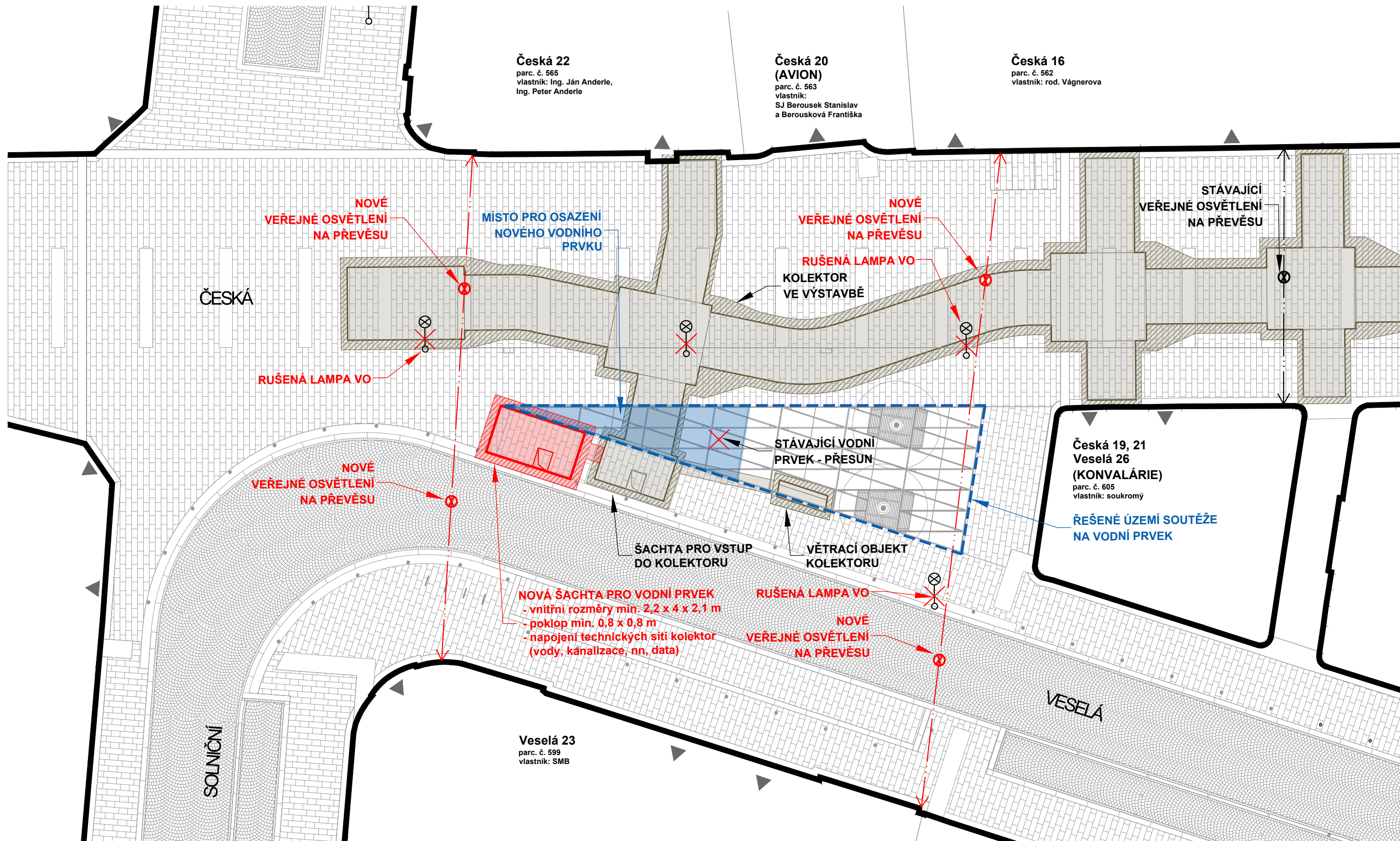
SCHÉMA KOORDINACE STAVBY KOLEKTORU S VODNÍM PRVKEM
