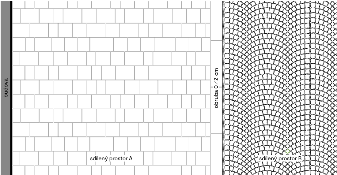
obr. 94 sdílený prostor A — dlažební desky kamenné [B.2.2.a] sdílený prostor B — štipané kostky kamenné [B.2.3.b]
